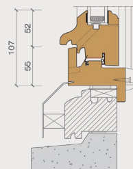
Pose en neuf avec aile intérieure rapportée
