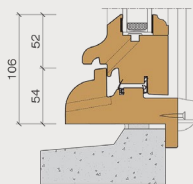
Pose en neuf avec rejingot Intégré sous appui
