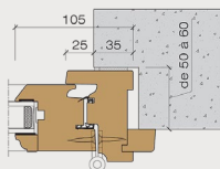
Pose en rénovation
