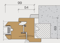
Pose en rénovation
